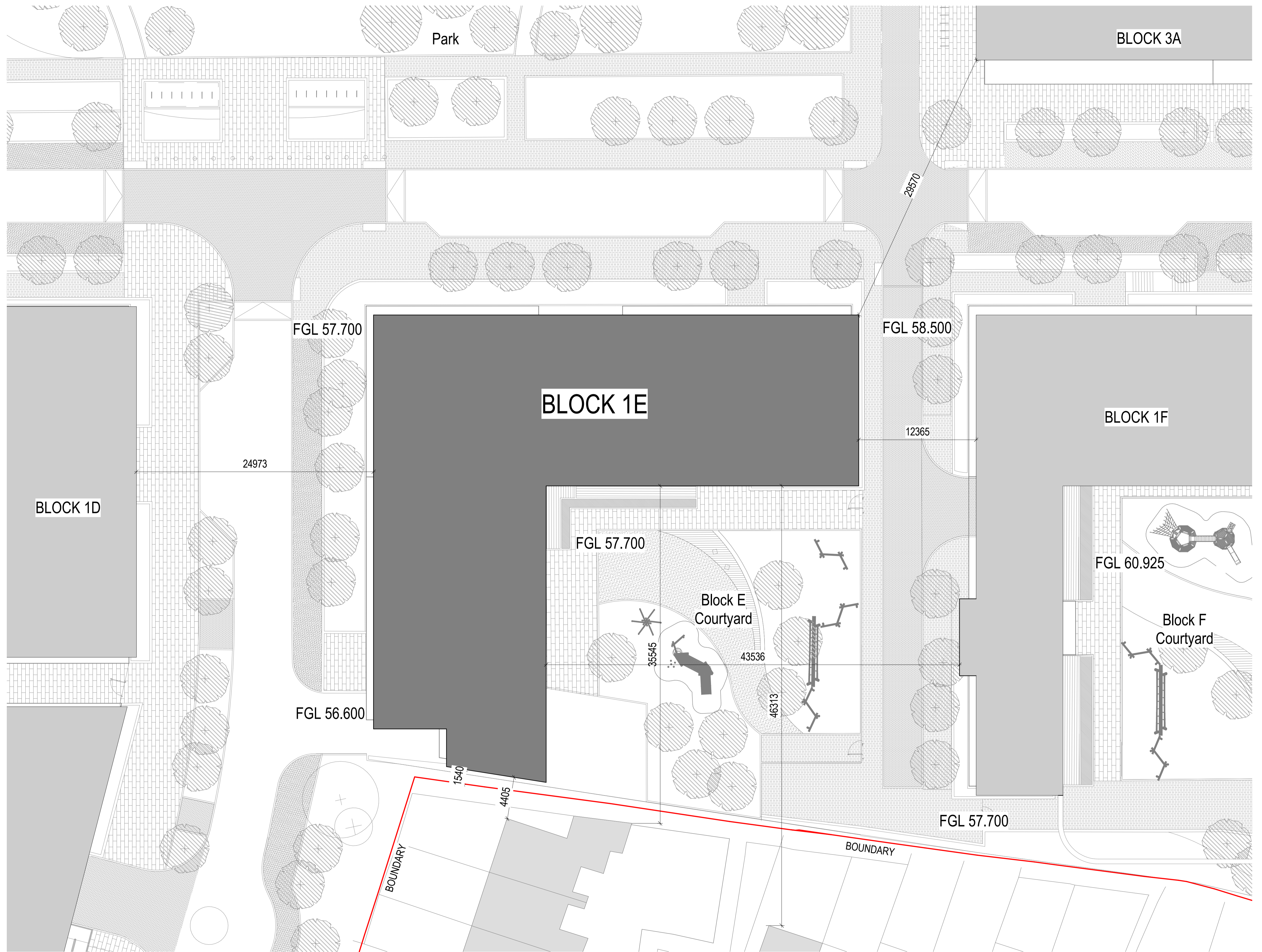
1 Block 1E_Site Plan 1 : 200
