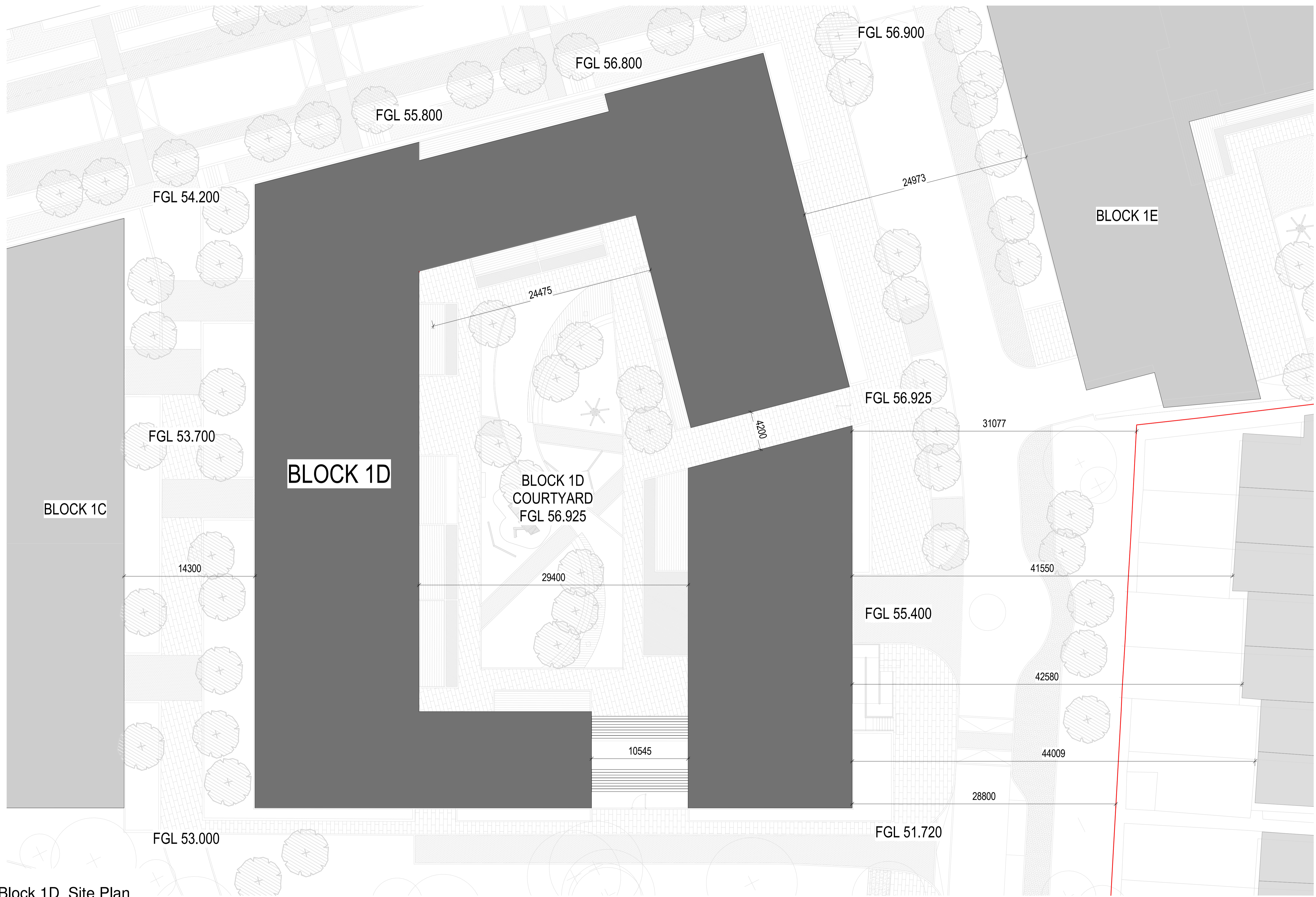
1 Block 1D_Site Plan 1 : 200
